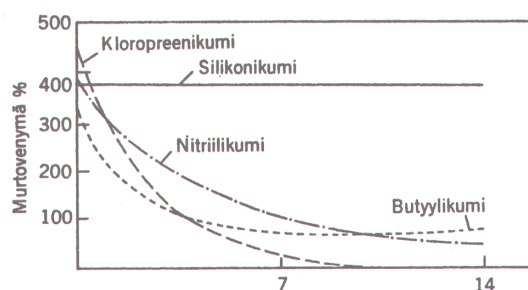
Murtovenymä 150°C lämpötilassa suoritetussa vanhennuskokeessa, mitattuna 25°C lämpötilassa.
