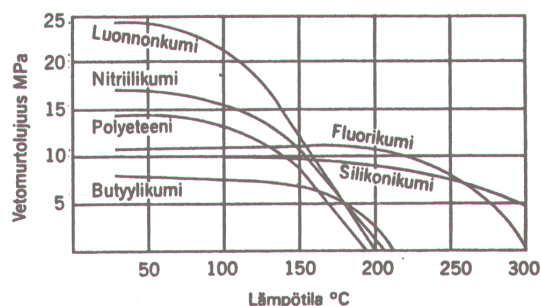
Vetomurtolujuus. Eri lämpötiloissa mitattu vetomurtolujuus 12 tunnin vanhennuskokeessa.
